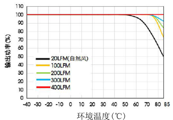
HSGS100-48S24S温度降额曲线( V_{in}=24V )
