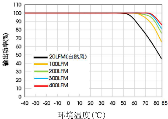
HSGS100-48S24温度降额曲线( V_{in}=24V )
