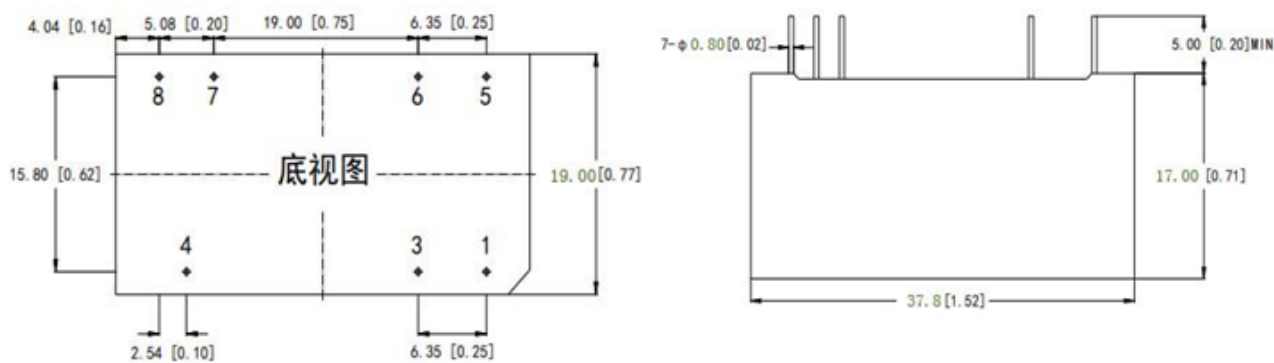
HSWD3W 系列机械尺寸图
